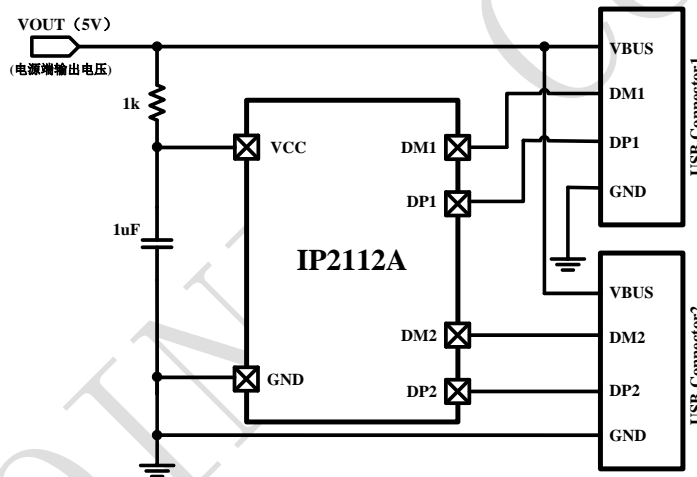
IP2112A 典型应用原理图
