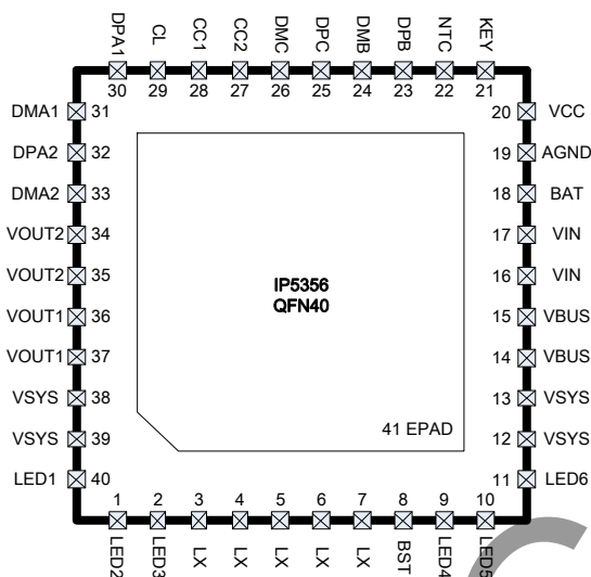
图 2 IP5356 引脚图
