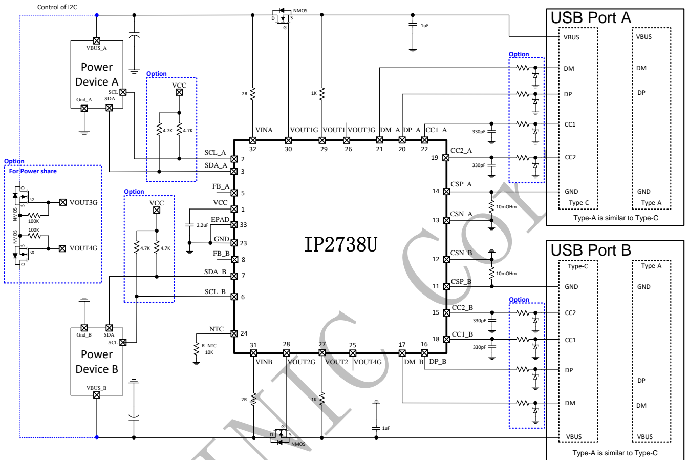
图 3. 双路独立 I2C 接口控制典型应用原理图
