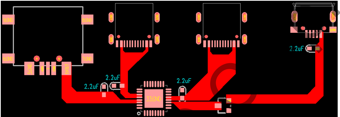
图 19 VOUT/VBUS1/VBUS2 电容位置
