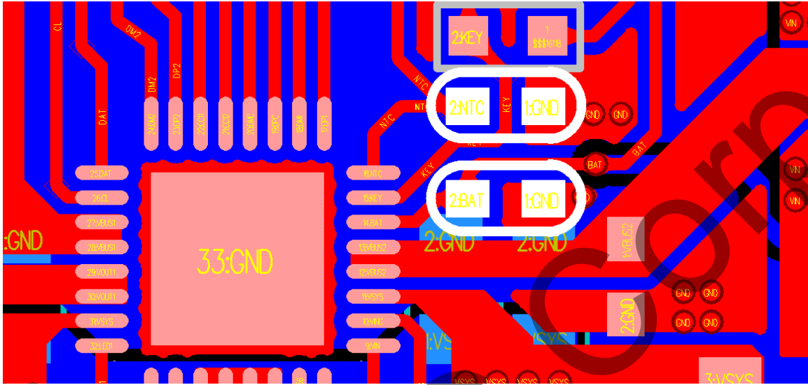
图 21 BAT/NTC 电容位置
