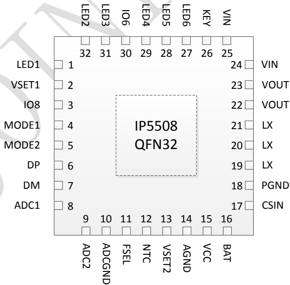
图 2 IP5508 引脚图
