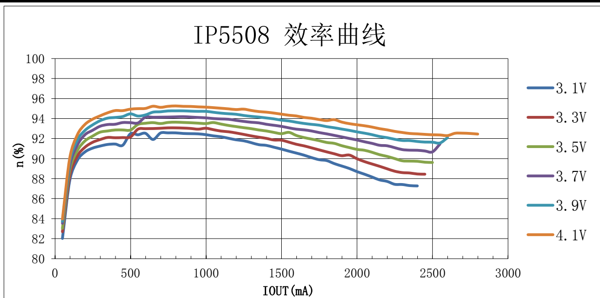
图4 IP5508 升压效率图
