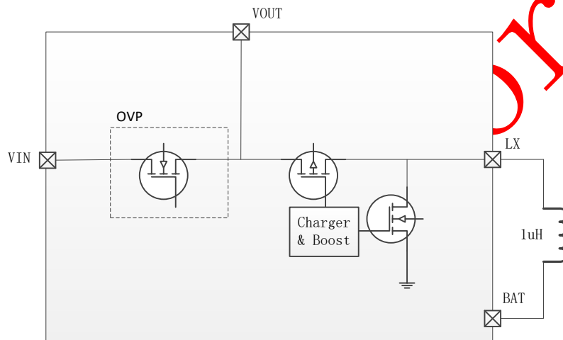
图6 IP5427 路径管理示意图
