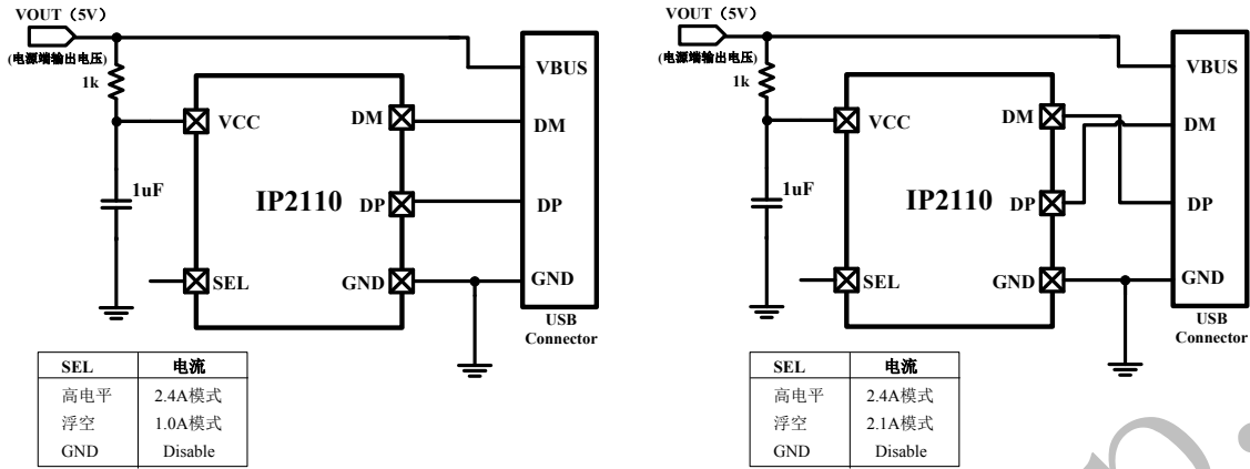
IP2110 典型应用原理图
