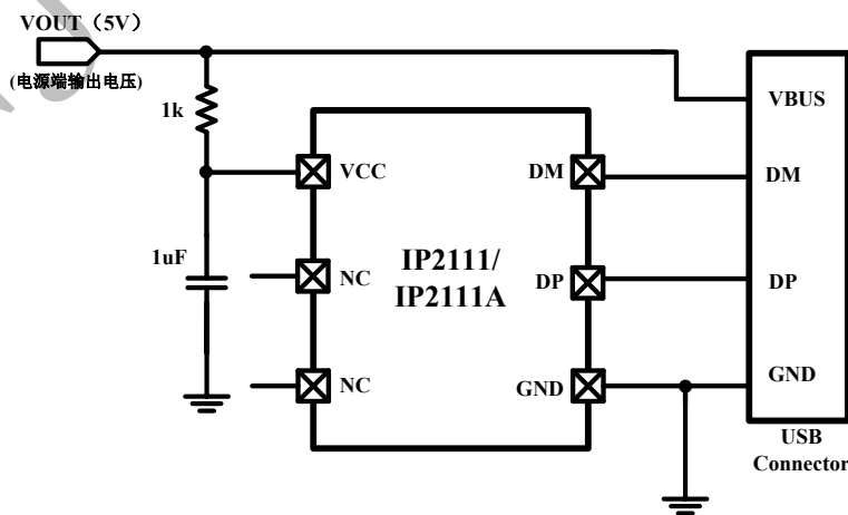
IP2111, IP2111A 典型应用原理图
